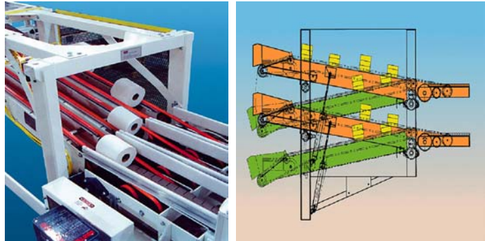
2 : 3 VERTICAL SWITCH
